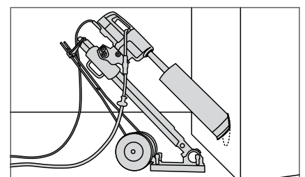
Boren onder een hoek.
