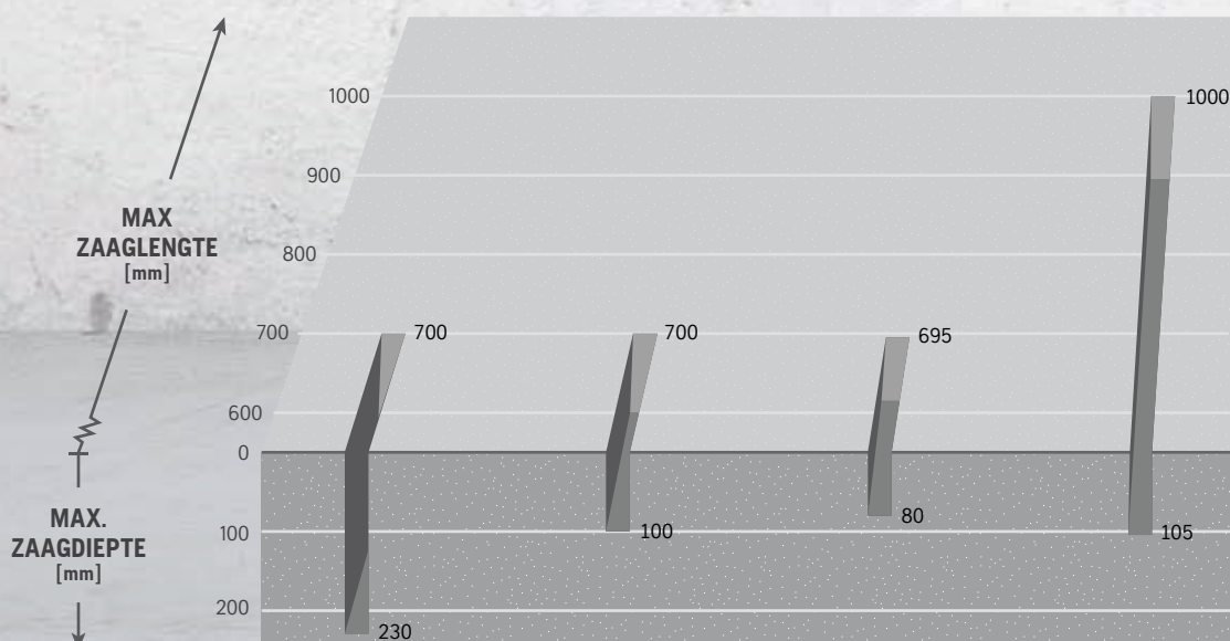
TS 400 F
