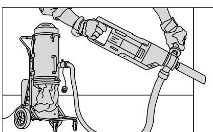
Droog boren uit de hand.
