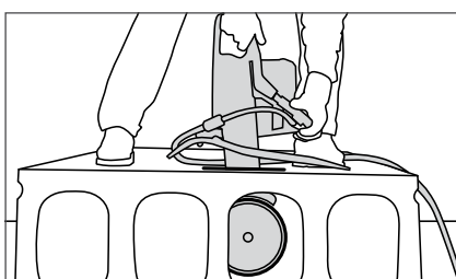
Zagen van gestort beton.
