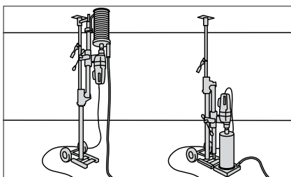
Verticaal boren, omhoog en omlaag.
